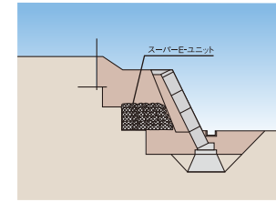
■ 土留め壁裏込材 湧水の多い法面の排水槽として使用
